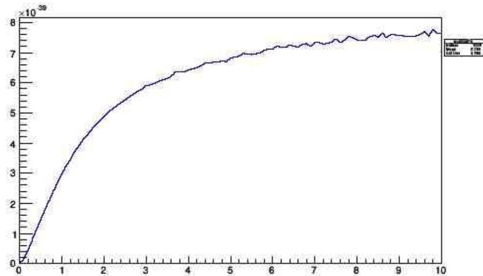
positron-Iron
